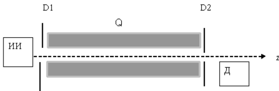
Рис. 3. Ионно-оптическая схема анализатора:
