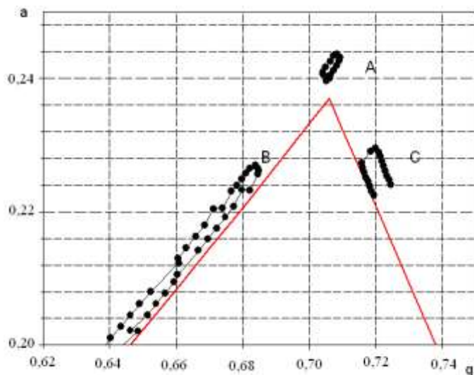
Рис. 6. Острова стабильности А, В и С, определенные экспериментально
