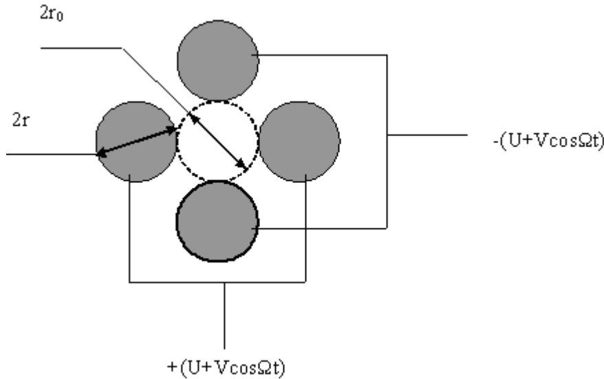
Рис 2. Схема питания электродов фильтра масс
