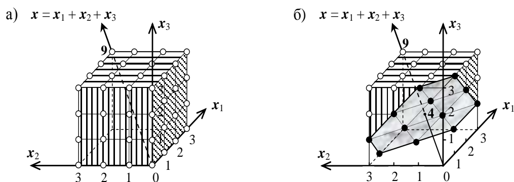
Рис. 6. Координатное представление возможных итогов решения контрольной работы из трех задач стоимостью три балла
