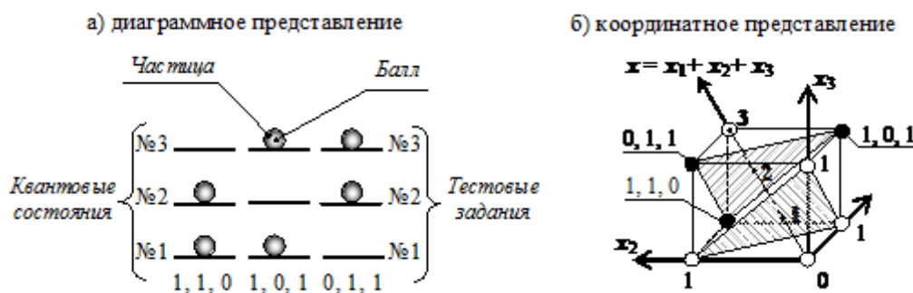
Рис. 1. Итоги тестирования учащихся набравших два балла за тест из трех заданий стоимостью один балл, в диаграммном и координатном представлениях
