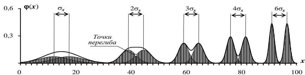
Рис. 9. Разрешение распределений \varphi(x) при различной полуширине, характеризуемой значением K\sigma_x = 0,5\sigma_x, \sigma_x, 1,5\sigma_x, 2\sigma_x, 3\sigma_x
