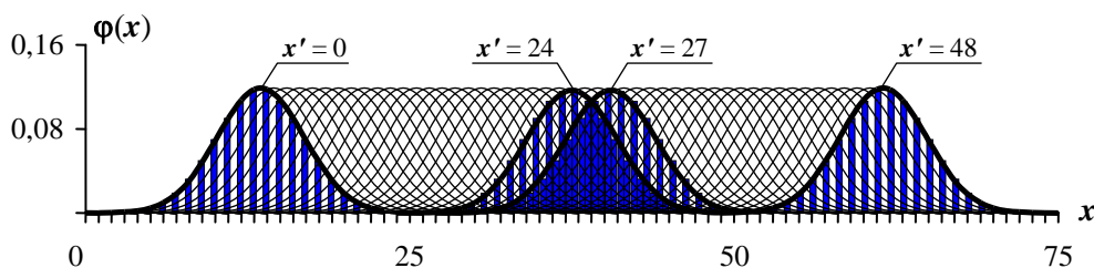
Рис. 8. Проблема введения спектральных характеристик контрольной работы при k = 16 , n = 25 , m = 3
