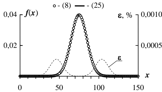
Рис. 5. Сравнение распределений f(x) (25) при m = 6, n = 25, k = 9, n - k = 16
