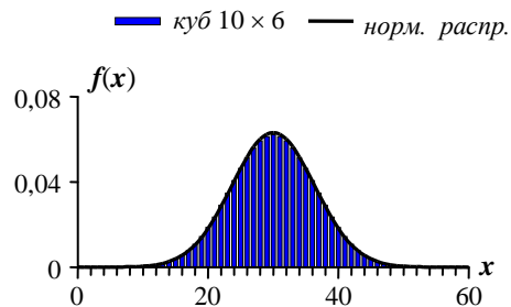
Рис. 3. Сравнение распределения точек вдоль диагонали в решетчатом кубе с нормальным распределением (8) при разной размерности куба n
