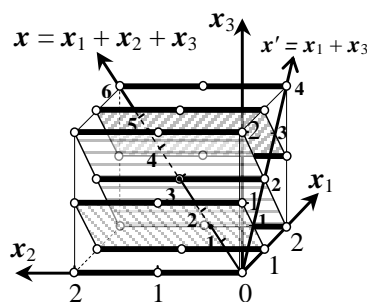
Рис. 4. Группировка точек решетчатого куба ( m = 2, n = 3 ) по плоскостям, нормальным к диагонали одной из граней
