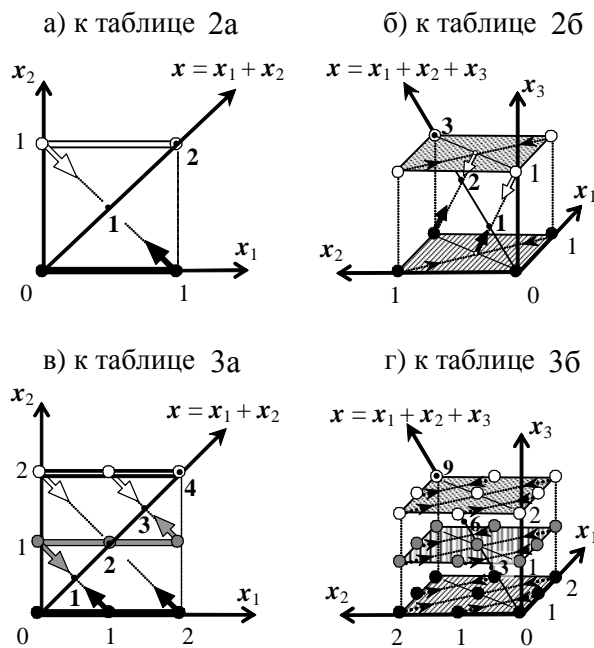
Рис. 2. Геометрическая интерпретация расчета распределения точек вдоль диагонали (вдоль оси 0x ) в решетчатом квадрате и решетчатом кубе при m = 1 (а,б) и m = 2 (в,г)
