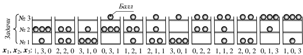
Рис. 7. Диаграммное представление возможных итогов решения контрольной работы из трех задач стоимостью три балла, когда испытуемый набирает за их решение четыре балла
