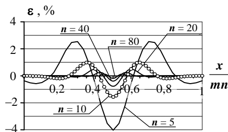
Рис. 3. Сравнение распределения точек вдоль диагонали в решетчатом кубе с нормальным распределением (8) при разной размерности куба n
