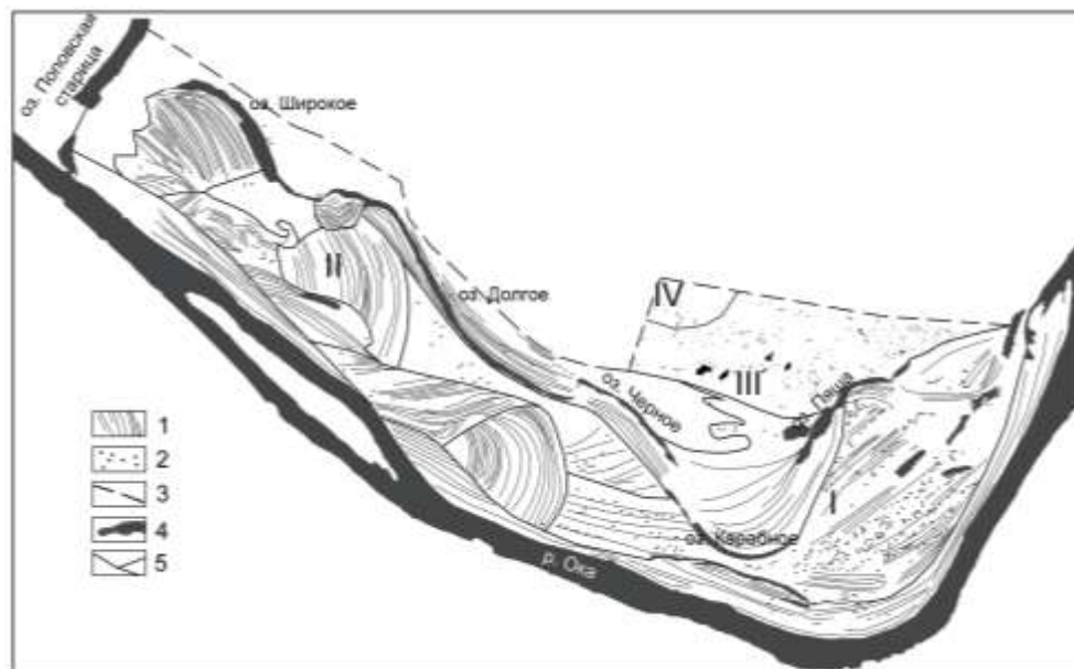
Рис. 1. Некоторые особенности геоморфологического строения территории Сосновского заказника
