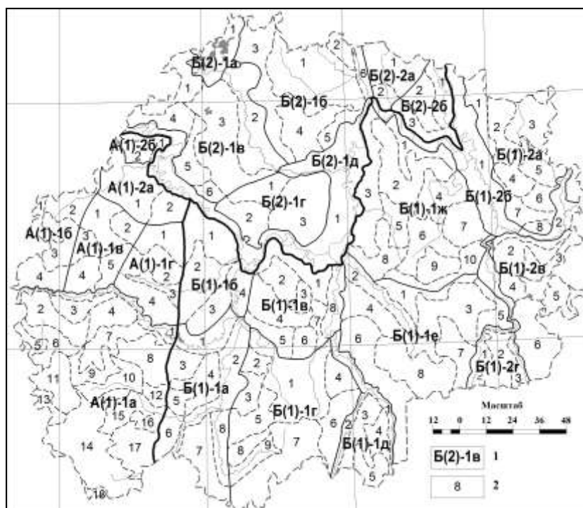
Рис. 2. Геоморфологическое районирование территории Рязанской области 1 – индексы подрайонов; 2 – номера местностей; линиями показаны границы разных таксонов геоморфологического районирования
