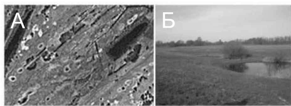
Рис. 4. Изображение западин, нанизанных на межгривные понижения параллельно-гривистых пойм на космоснимке (А) и на местности (Б)
