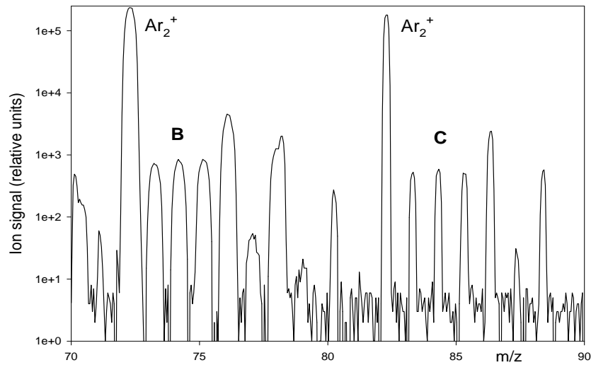
Рис. 6. Масс-спектр ионов аргона ( ^{80}\text{Ar}_2^+ ) и его изотопов, полученный при сканировании через два острова B и C при q' = 3,6\% . Энергия ионов равна 5 eV. \omega = 9/10 \Omega = 2,25 MHz, V' = 64 V, и V = 1254 V( p-p ) [15]
