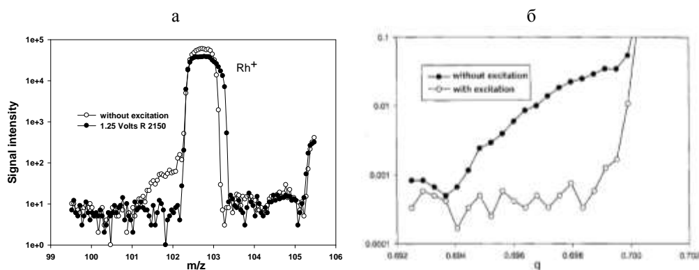
Рис. 7. (а) – устранение «хвоста» массового пика ионов ^{103}\text{Rh}^+ с параметрическим возбуждением ( \nu = 9/10 и q' = 0,012 ) и без возбуждения [9]; (б) – расчет низкокассового хвоста пика в обычном режиме ( \lambda = 0,166576 ) и острове стабильности ( \lambda = 0,166666 , q' = 0,012 ) [13]
