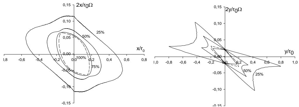
Рис. 4. Аксептанс КФМ в рабочей точке a = 0,233982 , q = 0,704396 при параметрах: d = 0,25 r_0 , z_f = 1,5 r_0 и n_f = 3 , определенных по 25-, 50-, 75- и 100-процентному уровням пропускания [24]
