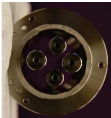
Рис. 8. Фотография электродов КФМ, формирующих 12-процентную гексапольную компоненту ( A_3 = 0,12 ); r_0 = 4,5 мм, \theta = 7,69^\circ , r_x = 5,9378 мм, r_y = 5,1692 мм [32]
