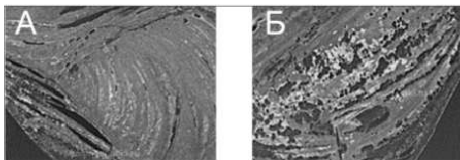
Рис. 3. Типы местностей в пойме: А – с преимущественным развитием сегментно-гривистых пойм; Б – с преимущественным развитием параллельно-гривистых пойм, осложненных округлыми западинами
