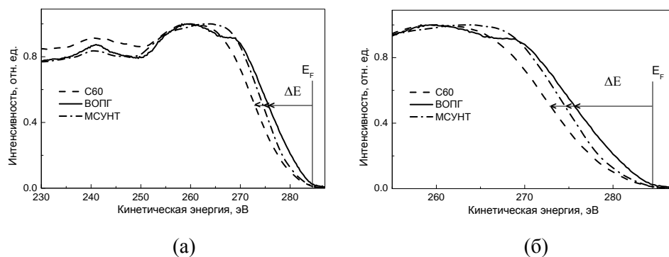
Рис. 1. с KVV спектры фуллерена C_{60} , ВОПГ и МСУНТ. Спектры аналогичны спектрам, представленным в [12]
